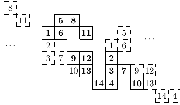
a standard tableau p
